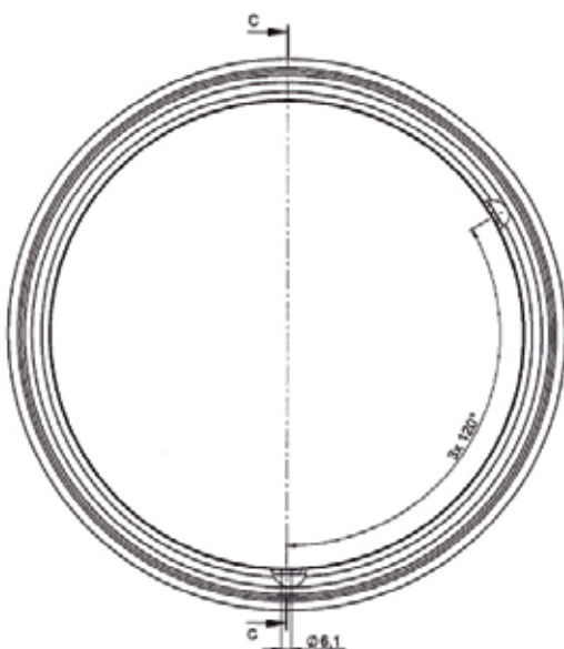
Beispiel Abdeckglas Siteco Große Glocke
